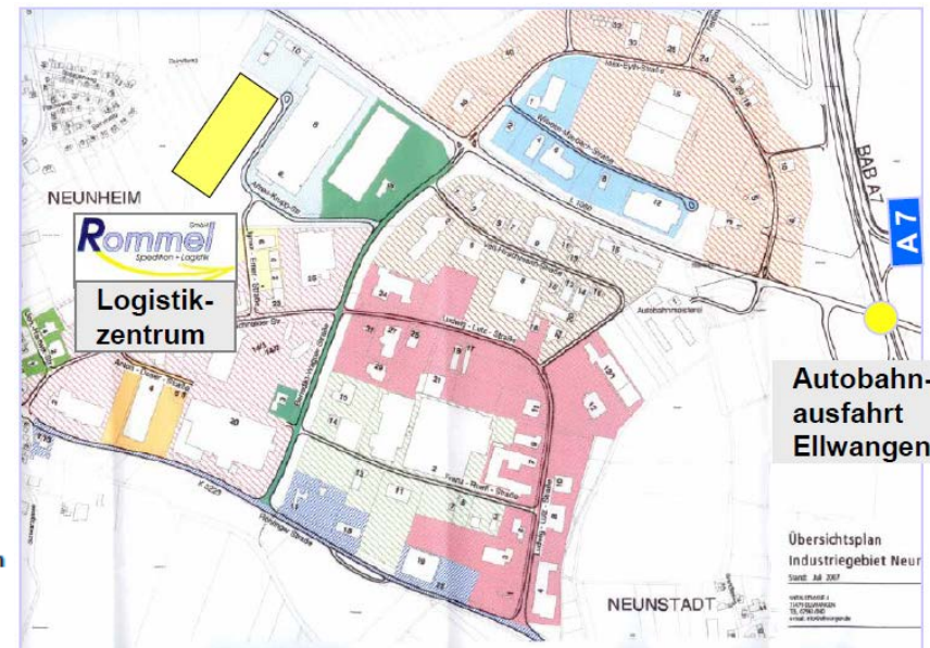
Grundstücksplan Industriegebiet Neunheim
